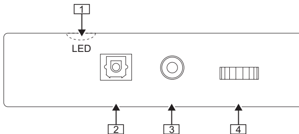
Abb. 3.1: Vorderseite UCA202
