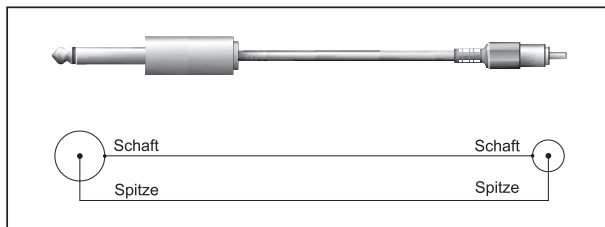
Abb. 5.2: Die Verdrahtung eines MONO Adapters
