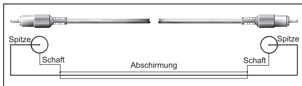
Abb. 5.1: Die Verdrahtung eines Cinchkabels
