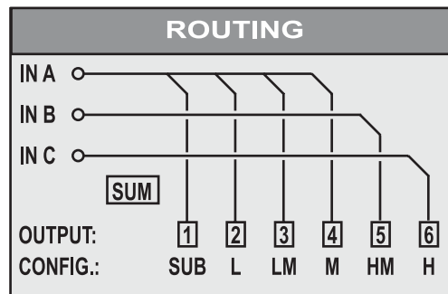
Abb. 6.10: Mono 4-Wege Betrieb plus 2 Monitore (pro Stereoseite)
