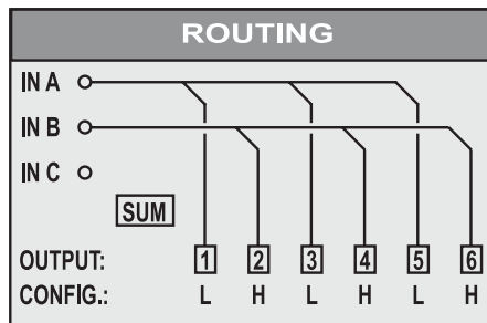
Abb. 6.8: Dreifache Stereo Delay-Line
