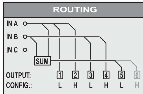
Abb. 6.2: Stereo 2-Wege-Betrieb plus Subwoofer
