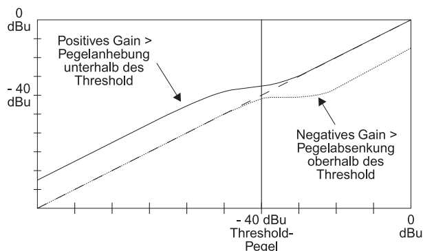
Abb. 4.36: Filterkurven bei Über- bzw. Unterschreiten des Threshold-Werts
