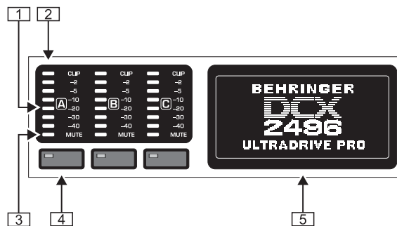
Abb. 2.1: Eingangs-LEDs und Display
