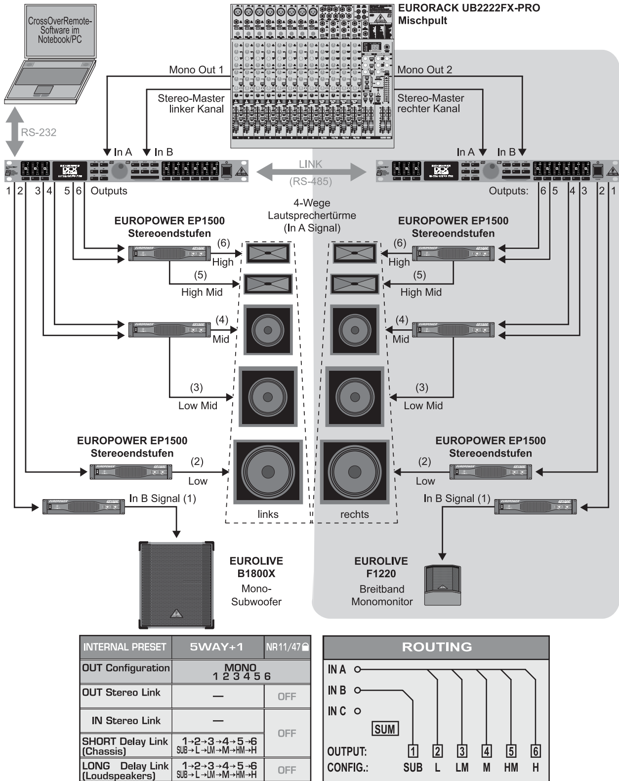
Abb. 6.11: Mono 5-Wege Betrieb plus 1 zusätzliches Monosignal (pro Stereoseite)
