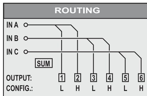
Abb 6.3: 3x2-Wege-Betrieb (LCR/Triple Bi-Amping)
