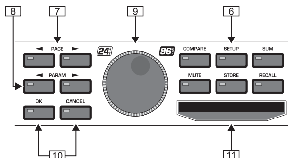
Abb. 2.2: Menü-Taster und Datawheel
