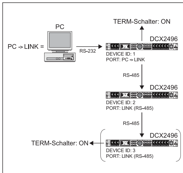
Abb. 4.30: Der PC -> LINK-Modus
