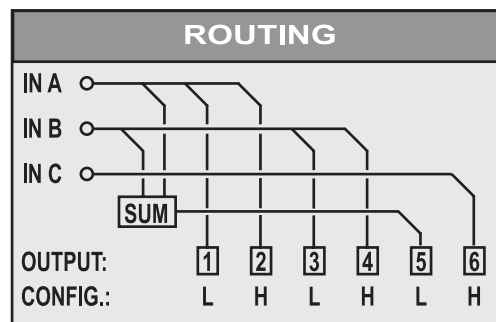
Abb. 6.6: Stereo 2-Wege-Betrieb plus Subwoofer und zusätzlicher Monitor
