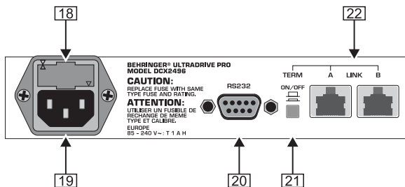
Abb. 2.4: Netzanschluss und RS-232/RS-485-Verbindung
