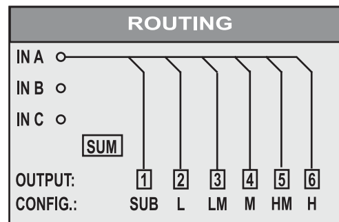
Abb. 6.7: Mono 6-Wege "Zoning" (Signalverteilermodus)
