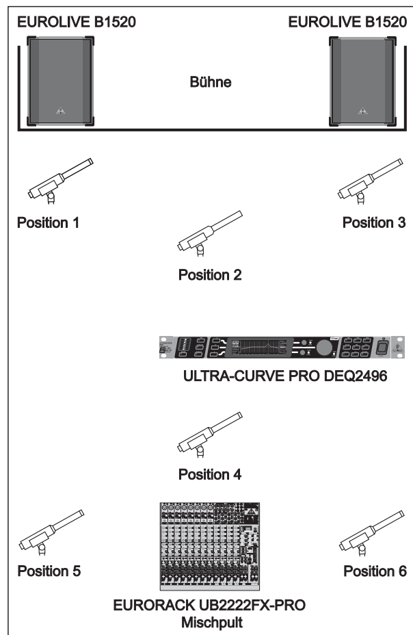
Abb. 4.2: Positionierung des Messmikrofons
