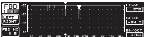
Abb. 3.8: Das FBD-Menü (Seite 1)
