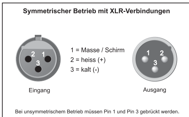
Abb. 5.1: XLR-Verbindungen
