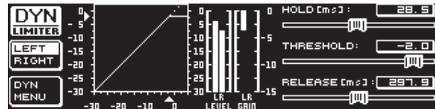
Abb. 3.15: Das LIMITER-Menü
