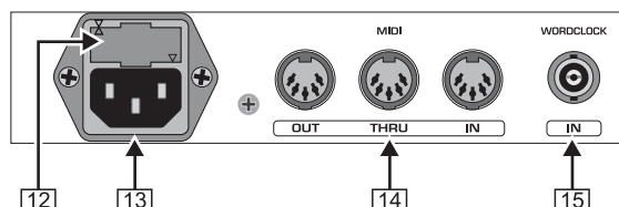
Abb. 2.4: Netzanschluss, MIDI- und Wordclock-Verbindungen
