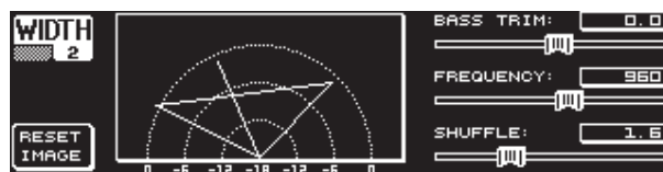
Abb. 3.12: Das WIDTH-Menü (Seite 2)
