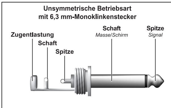
Abb. 5.2: 6,3-mm-Monoklinkenstecker
