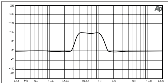
Abb. 3.18: Grafischer Equalizer mit Frequenzgangkorrektur (TRUE RESPONSE)
