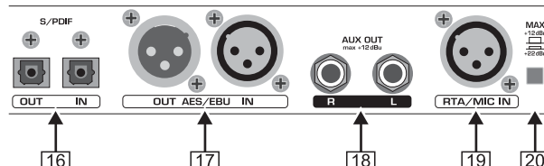
Abb. 2.5: Digitalschnittstellen und RTA-Mikrofoneingang
