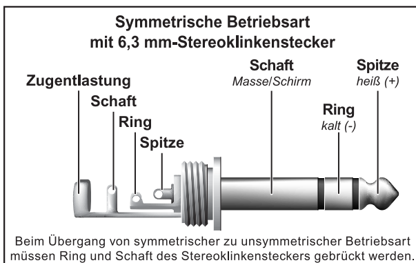
Abb. 5.3: 6,3-mm-Stereoklinkenstecker
