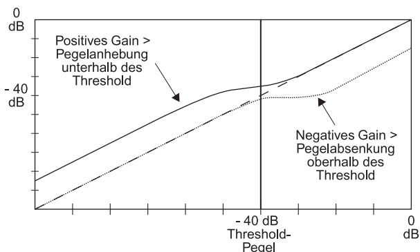
Abb. 3.7: Filterkurven bei Über- bzw. Unterschreiten des Threshold-Werts
