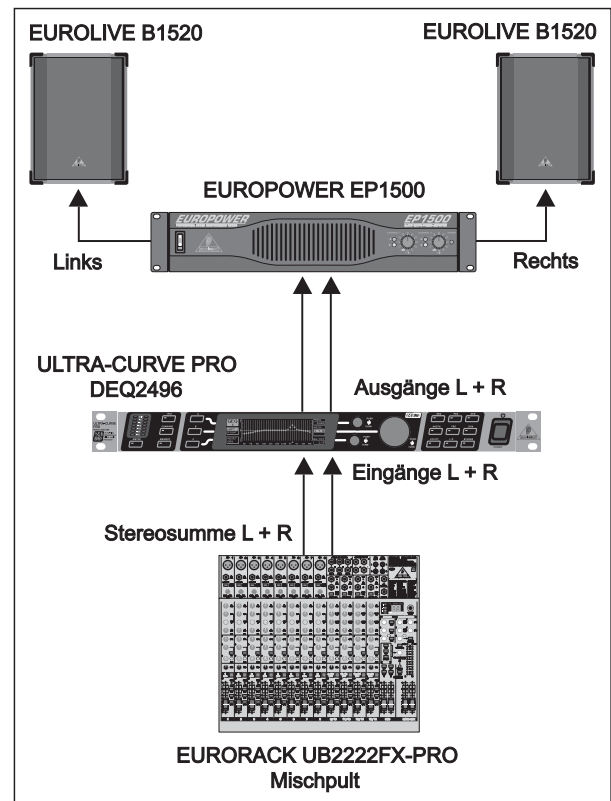
Abb. 4.1: Der ULTRA-CURVE PRO als Summen-Equalizer
