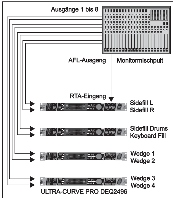
Abb. 4.3: Mehrere ULTRA-CURVE PRO in einer Monitoranlage
